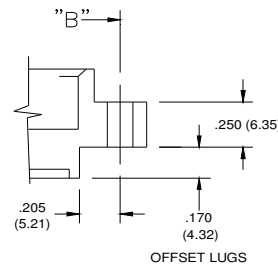
OFFSET LUGS
