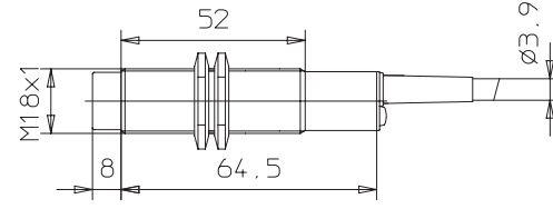
E2EL-X15M□ 2M
