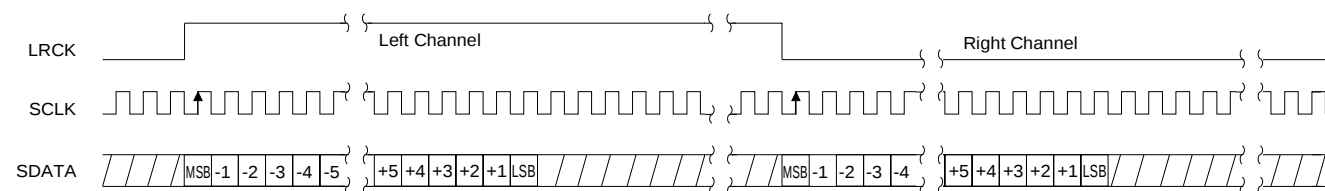
Figure 21. CS4341 Format 1 (I 2 S)
