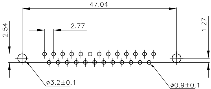
P.C.B. LAYOUT
