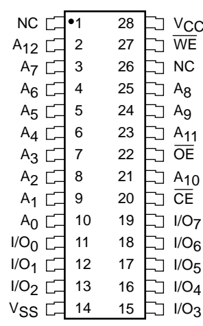
SOIC Package (J, K)
