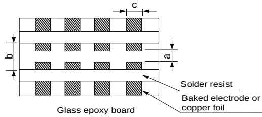
Fig.3 (in:mm)
