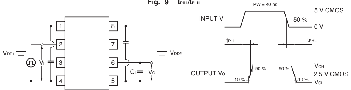
Fig. 9 t_{PHL}/t_{PLH}
