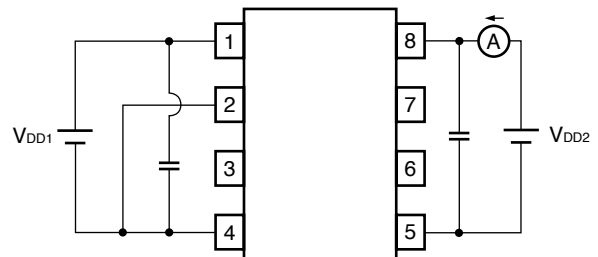
Fig. 6 I_{DD2L}
