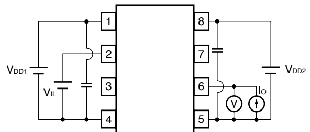
Fig. 8 V_{OL}
