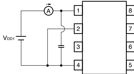
Fig. 1 I_{DD1L}
