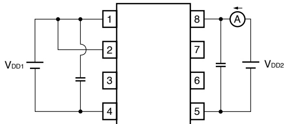
Fig. 5 I_{DD2H}
