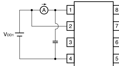
Fig. 2 I_{DD1H}
