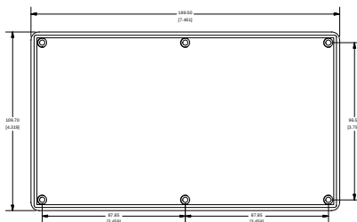
BOTTOM OF LID
