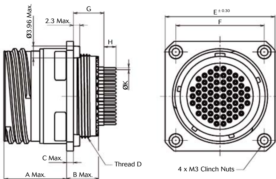
Jam nut receptacle (type 34)
