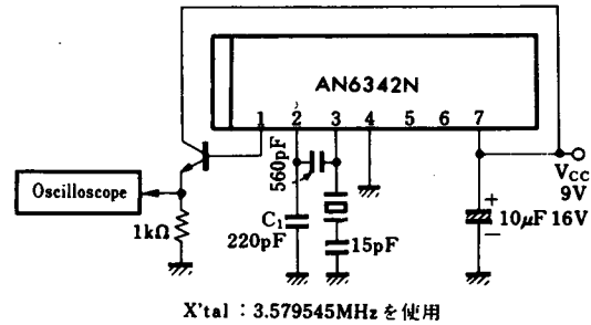
Test Circuit 2 (V O )
