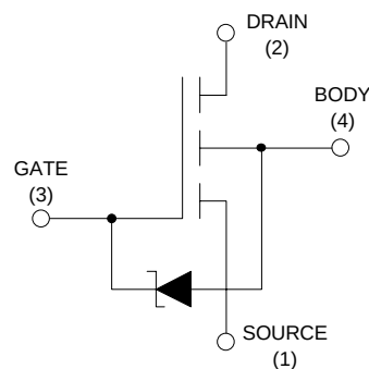
SOT-143
