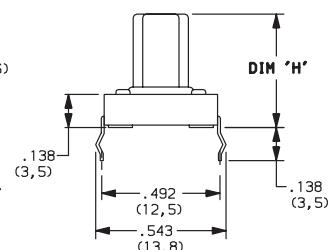
PTS125SM12 SPST
