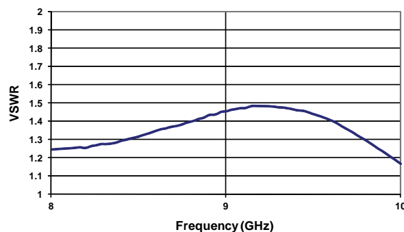
VSWR ( 8-10 GHz )
