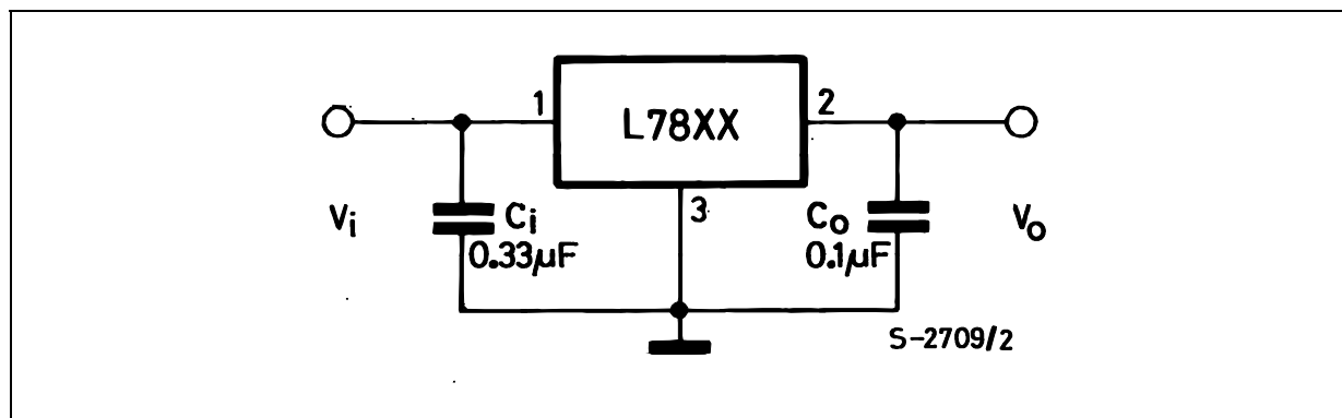
Figure 1 : DC Parameter
