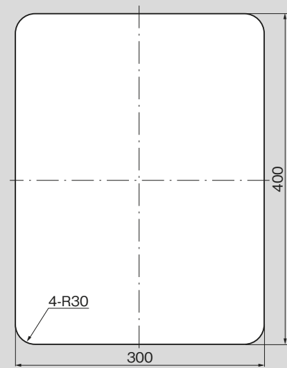
パネル穴明け寸法 Panel drilling dimensions
