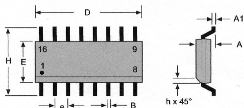
HMC1022—16-Pin SOIC
