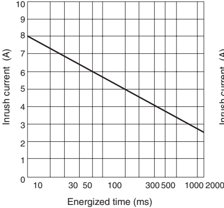
G3R-ODX02SN-UTU
