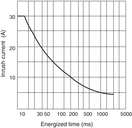
G3R-OA202SZN-UTU/OA202SLN-UTU
