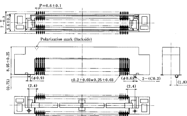
[FX8C- **/ **S11-SV5J]
