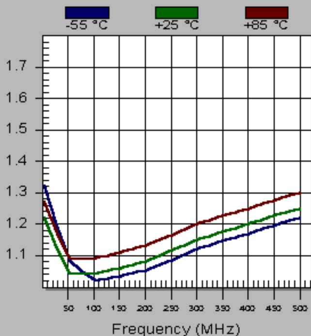
TM6523 Output VSWR
