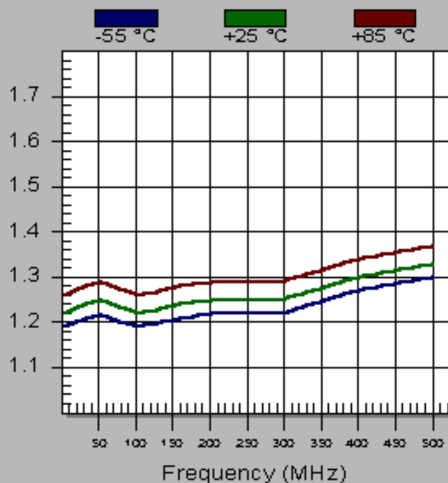
TM6523 Input VSWR
