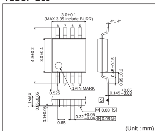
TSSOP-B8J
