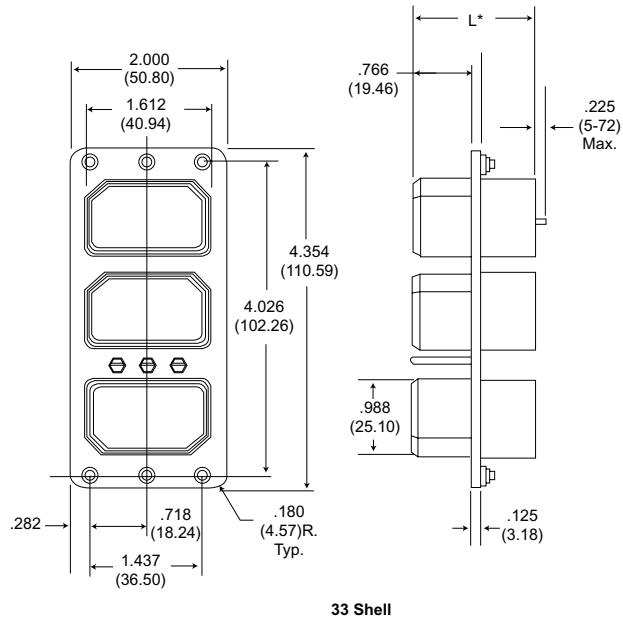
33 Shell
