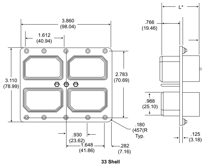
33 Shell
