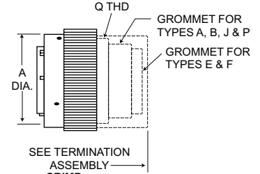
KPSE06/MS3126
