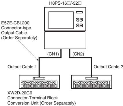
Output Cable 1
