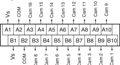
Output Cable 1
