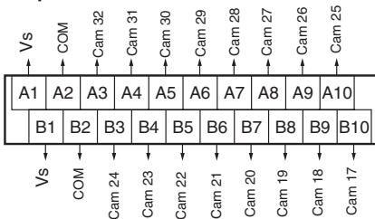
Output Cable 2
