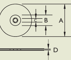
Reel Dimensions
