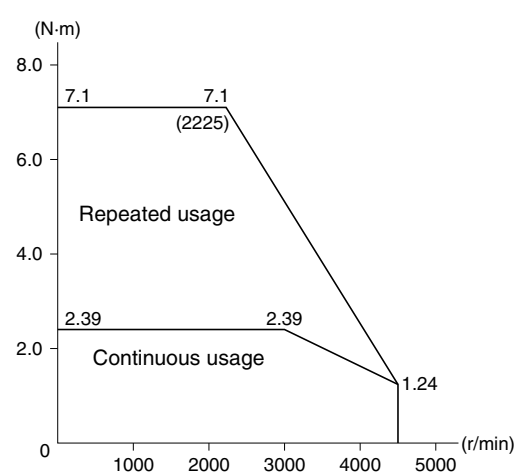
R7M-A75030 (750 W)
