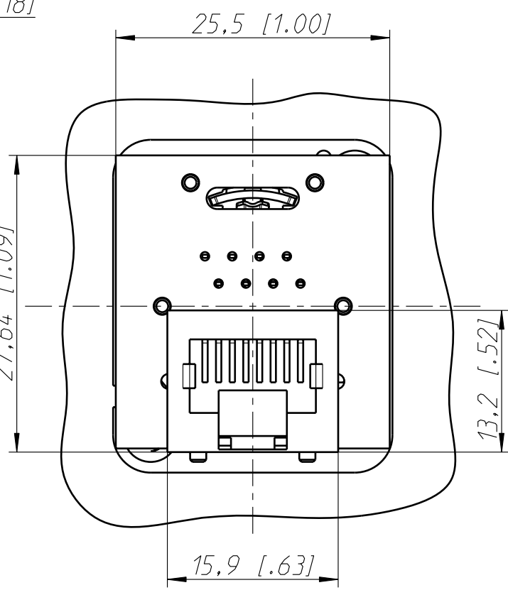
Frontplattenausschnitt (Rueckseite) Panel cut out (rear side)
