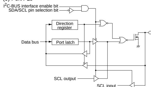
(9) Port P23
