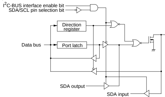
(8) Port P22
