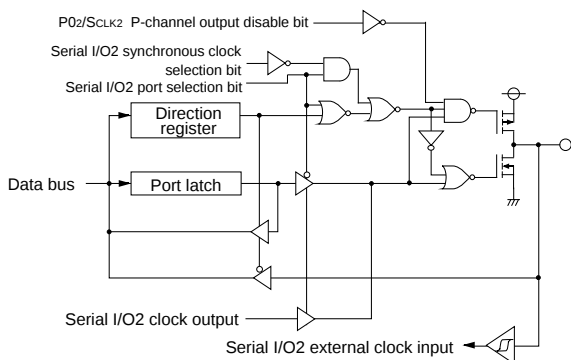
(3) Port P02
