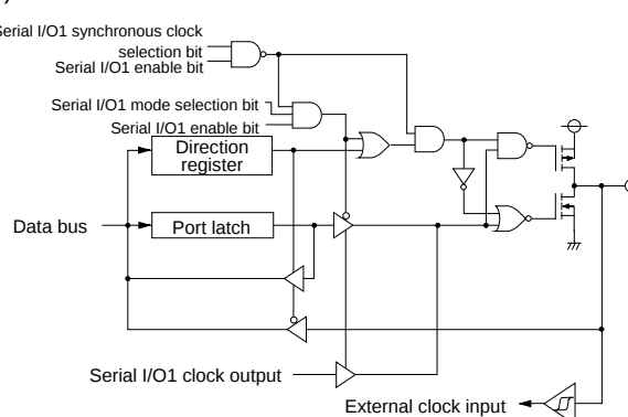
(12) Port P26
