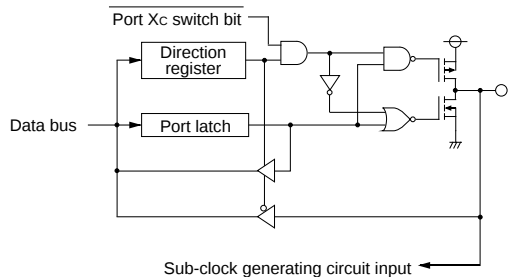
(7) Port P21
