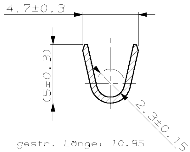
Schnitt: B-B
