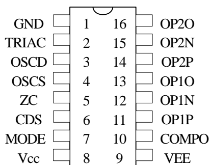
PT8A2647P/2647W
