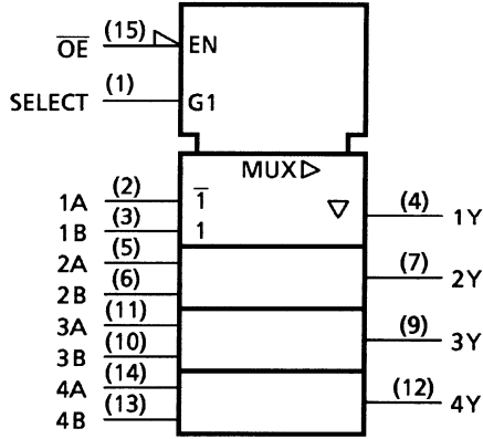
TC74AC257
