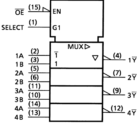
TC74AC258
