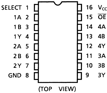
TC74AC257
