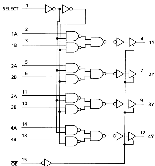
TC74AC258
