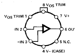
TO-99 (J-Suffix)
