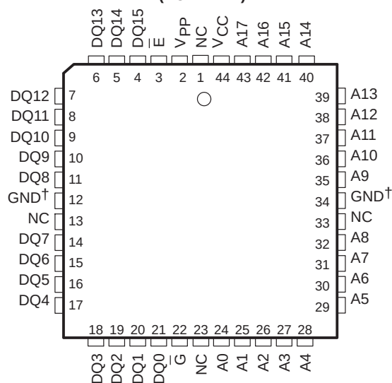
PIN NOMENCLATURE
