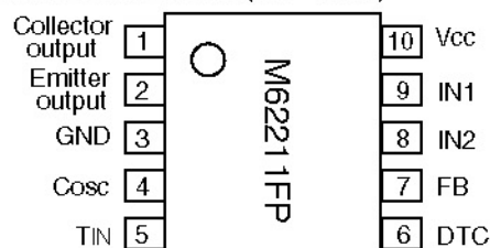
OUTLINE 10P2N-A
