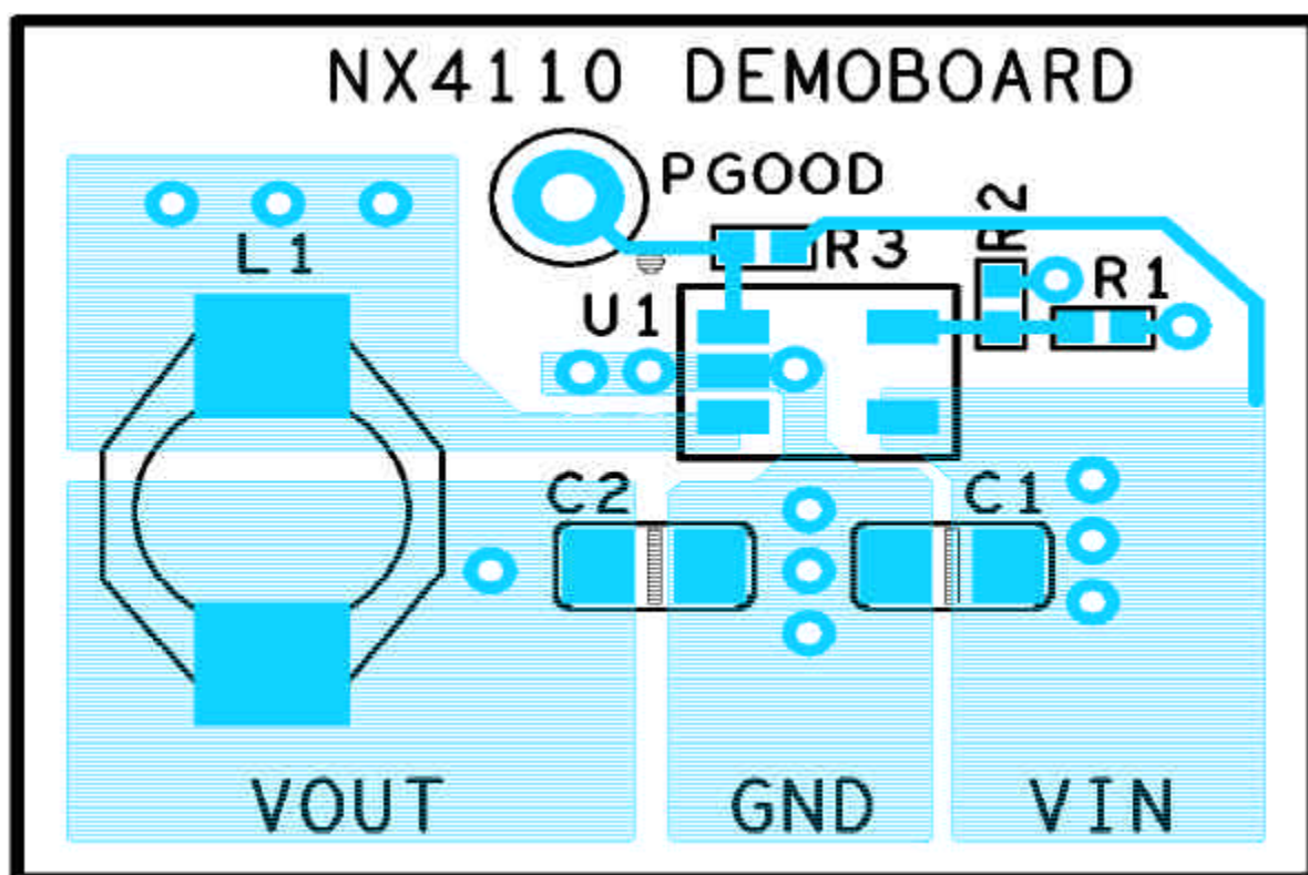
Fig. 20- Top layer
