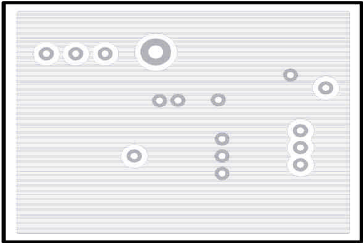
Fig. 21 - Gound layer
