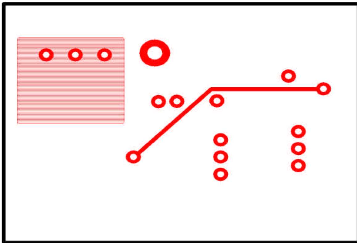
Fig. 23 - Bottom layer
