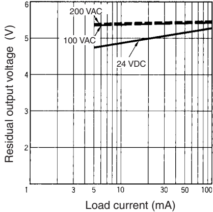
E2E-X□T1
