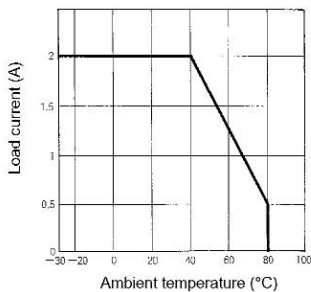
G3R-102□, G3RD-X02□, G3R-202□
