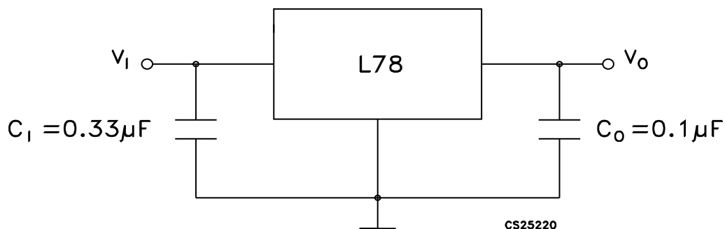
Figure 5. DC parameter
