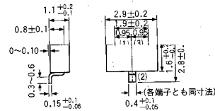
図5 SMT
