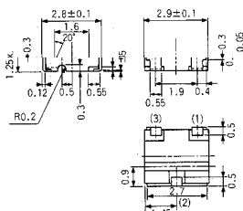
図4 MMT
