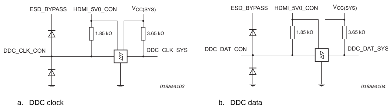
Fig 16. DDC circuit
