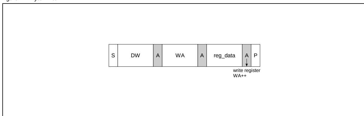
Figure 21. Byte Write
