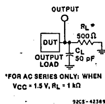
Fig. 5 - Test circuit.
