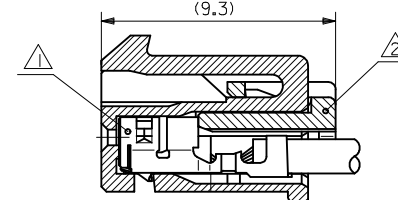
ターミナル及びリテーナー装着状態図 TERMINAL & RETAINER ASSEMBLY DRAWING
