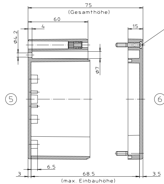
Zylinderschraube M4 x 24/10 ähnl. DIN EN ISO 7045
