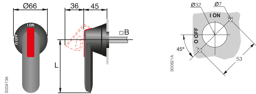
Door drilling for OH_ handles:
