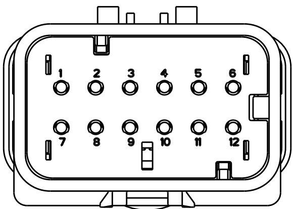
776438-2 SCALE 2:1
