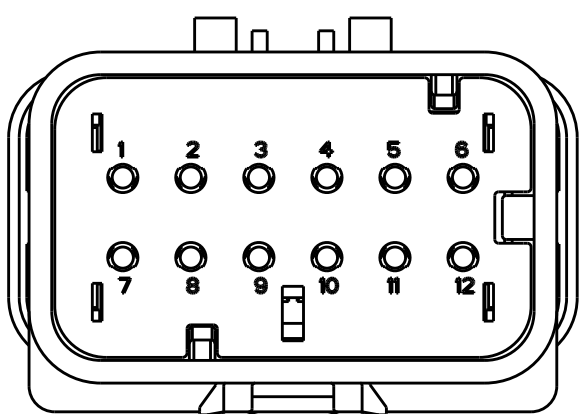
776438-3 SCALE 2:1
