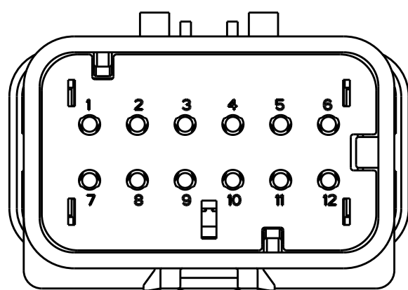
776438-4 SCALE 2:1
