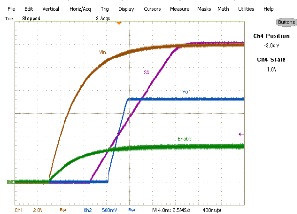
Fig. 7. Start up at 6A Load Ch 1 : V_{in} , Ch 2 : V_o , Ch 3 : V_{ss} , Ch 4 :Enable
