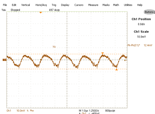
Fig. 10. Output Voltage Ripple, 6A load Ch 1 : V_o
