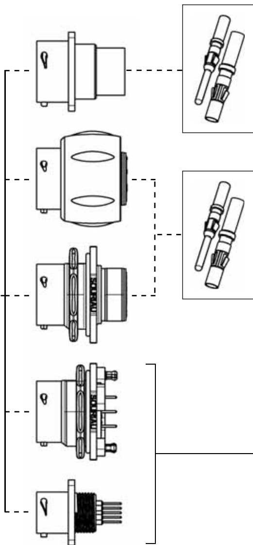
Receptacle
