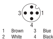
5 Pole/4 Wire
