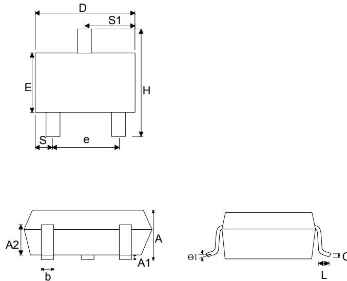
SOT-23-3
