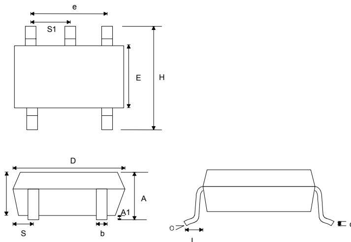
SOT-23-5
