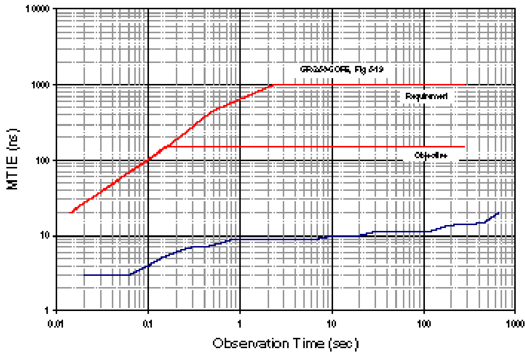
Phase Transients – MTIE
