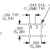
TS01ABE Horizontal Actuation SPDT
